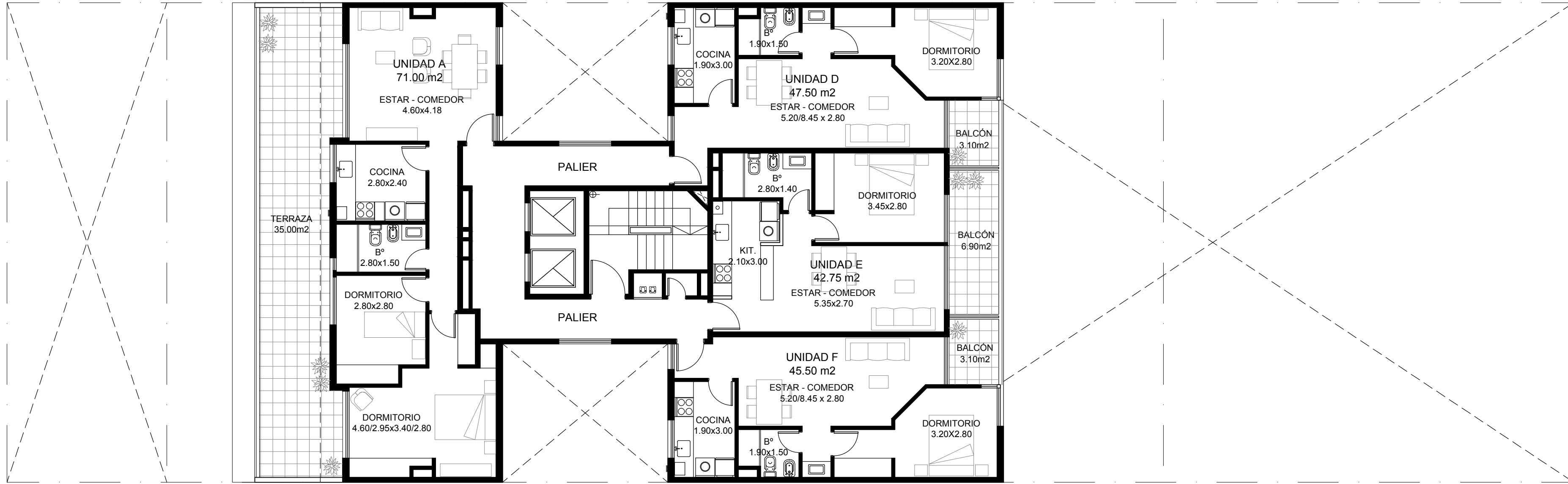
PLANTA 9° PISO 1:100
